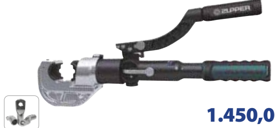
HZ-400 | 16 - 400 mm 2 Hidrolik Alüminyum ve Bakır Kablo Papuç Sıkma Pensesi
