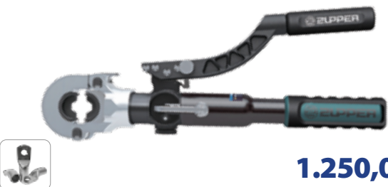
HZ-300 | 16 - 300 mm 2 Hidrolik Alüminyum ve Bakır Kablo Papuç Sıkma Pensesi
